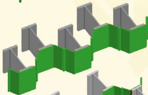
Рис. 2. Усиленная РШС.
